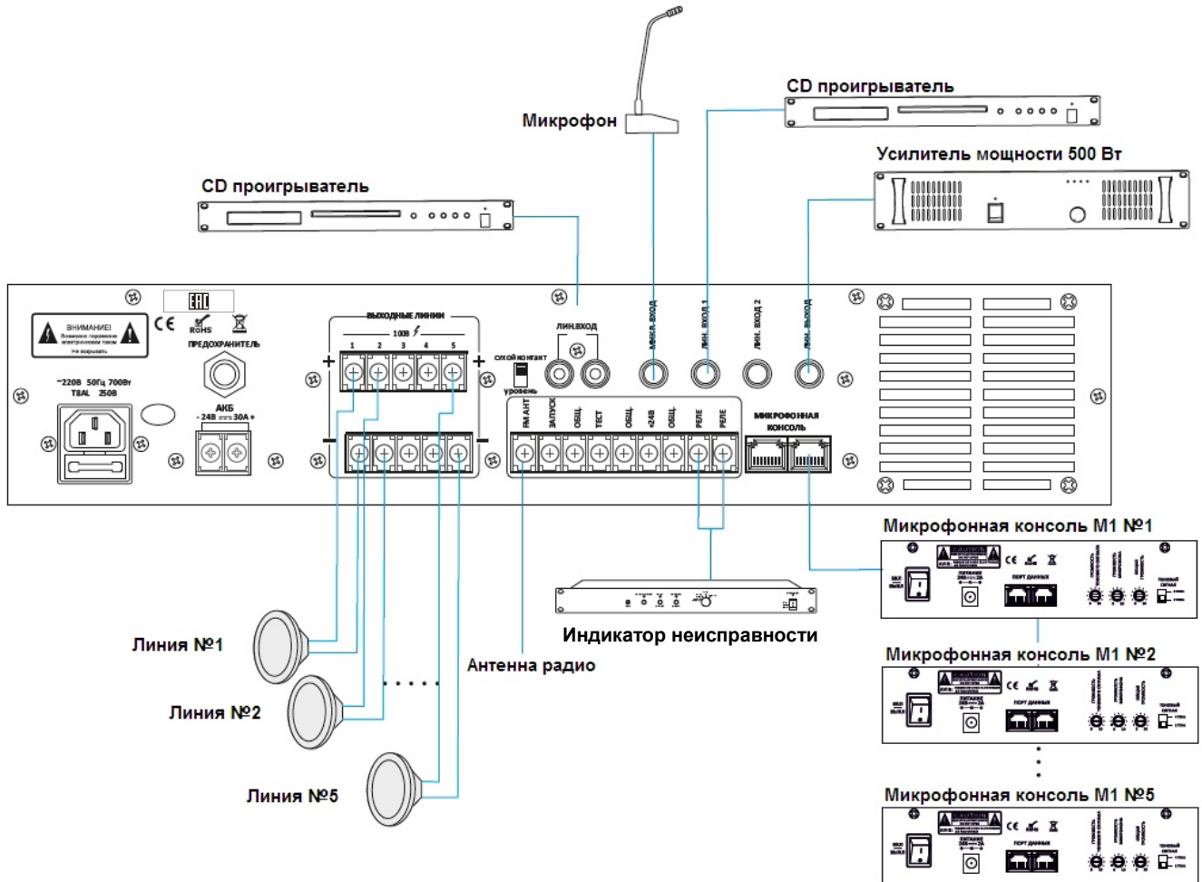
Рис. 2.1. Схема подключения
