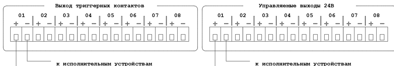
Рис. 3.1.6. Схема подключения внешних исполнительных устройств к LPA-DUO
