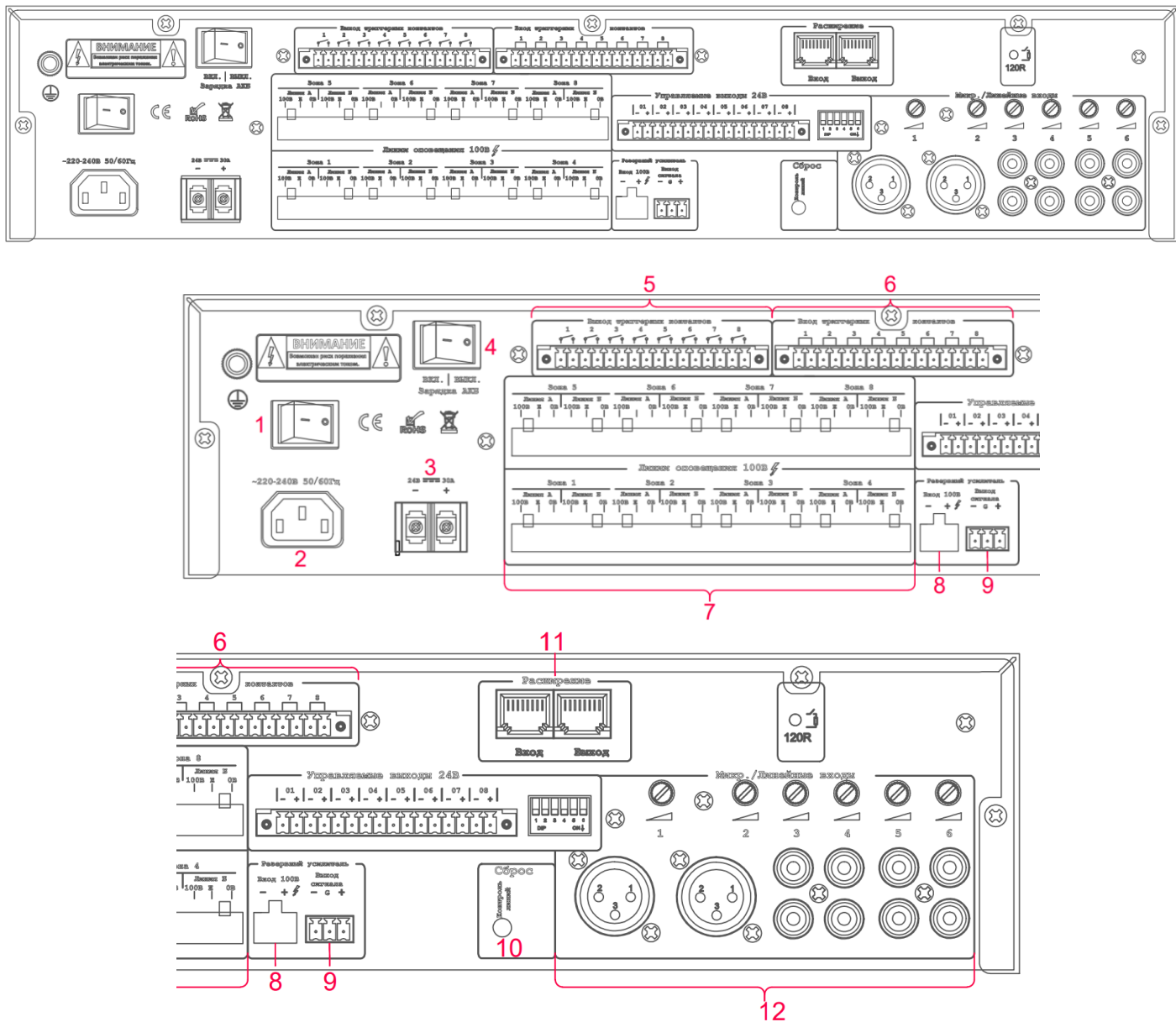
Рис. 2.2.3. Блок расширения LPA-DUO-S (задняя панель)
