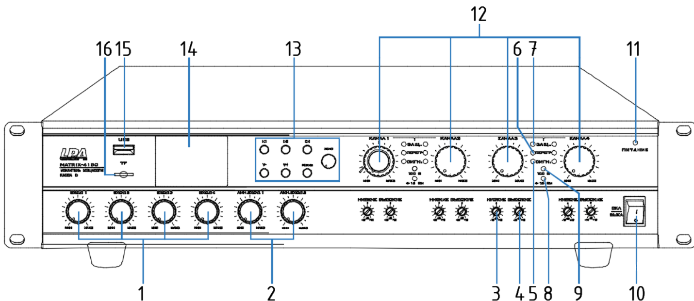
Рис.2.2. Передняя панель
