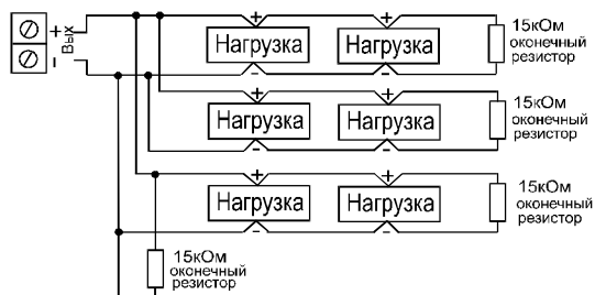
Рисунок 9б. Схема параллельного подключения трех (четырёх) линий нагрузок на выход управления
