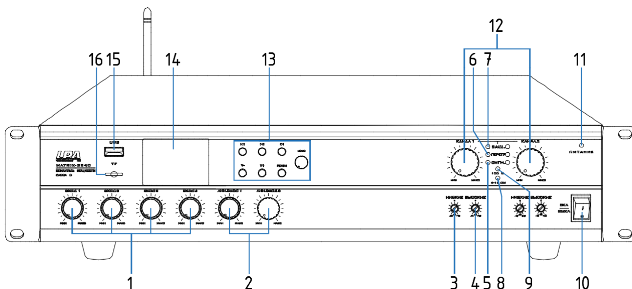
Рис.2.2. передняя панель
