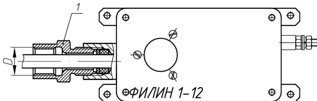
Рис. А.2.а Габаритный чертёж Оповещателей Филлин-1-12-БЗ (без звукового сигнала). Вариант со штуцером 1 для монтажа кабеля в металлорукаве. Остальные размеры и применяемые кабели см на рис. А.1.
