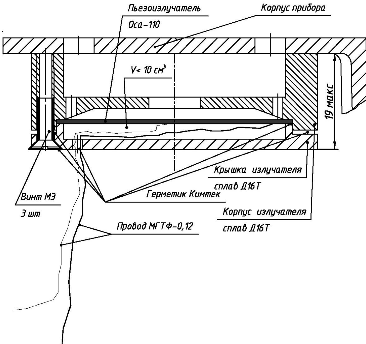
Рис. А.5 Рисунок звукового излучателя для Оповещателей Филин-1 и Филин-2
