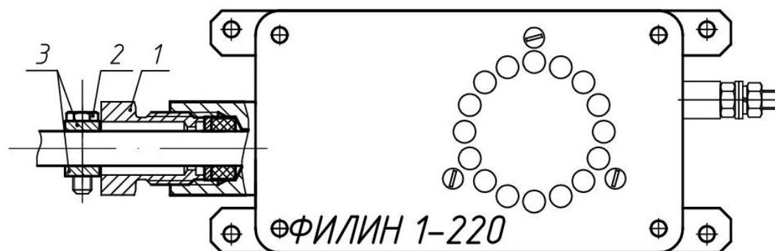
Рис. А.2.б Габаритный чертёж Оповещателей Филлин-1-220-БС (без светового сигнала). Вариант со штуцером для монтажа бронированного кабеля. Применяемый бронированный кабель – МКЭКШВнг(А)-хл 1x2x1 или МКЭКШВнг(А)-хл 2x2x1, или подобные негорючие. Остальные размеры см на рис. А.1.
