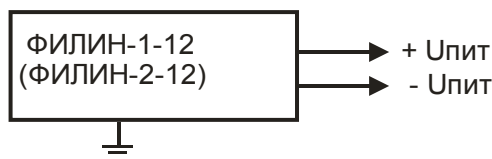
Рис. Б.1- Схема подключения Оповещателей модели ФИЛИН-1-12 и ФИЛИН-2-12. Положительный вывод кабеля отмечен красным цветом. Диапазон подключаемых напряжений 10,6... 28,0 В постоянного напряжения
