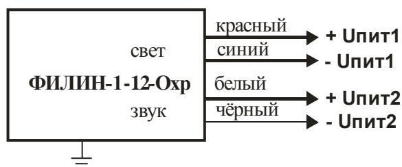
Рис. Б.3 Схема подключения Оповещателей модели ФИЛИН-1-12-Охр с отдельным питанием электрических схем звукового и светового сигнала. При подаче напряжения Упит1 включается световой сигнал, Упит2 – звуковой сигнал. Диапазон подключаемых напряжений 10,6...28,0 В постоянного напряжения. Электрические схемы светового и звукового сигналов гальванически развязаны.
