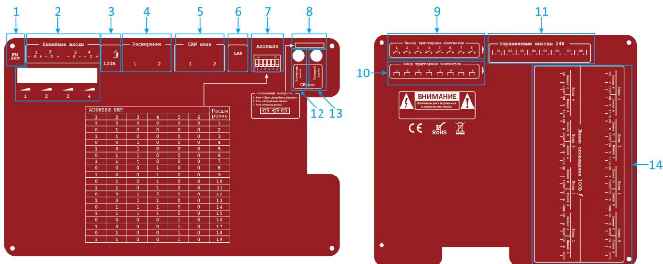
Рис. 2.2. Контроллер системы LPA-PRESTA-8 (внутренняя панель)
