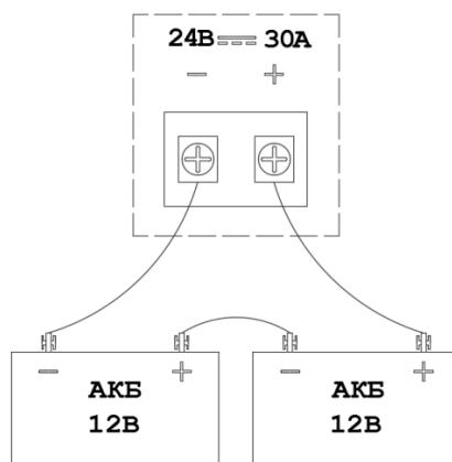
Рис. 3.1. Схема подключения АКБ к LPA-PRESTA-8
