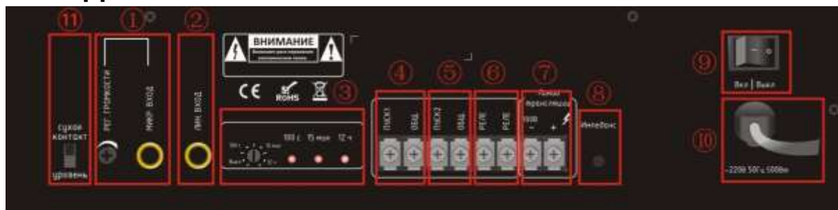
Рис. 1.3. Задняя панель LPA-MINI300
